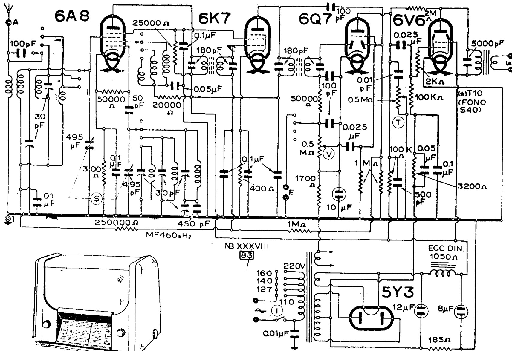
WATT RADIO - MOD. « SUPER STELLA 42 »
